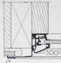
SIDE JAMB
