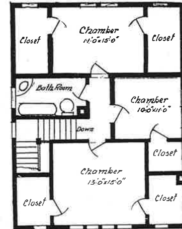
Second Floor Plan. V. W. Voorhees Archt
